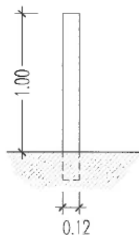
prospetto laterale
